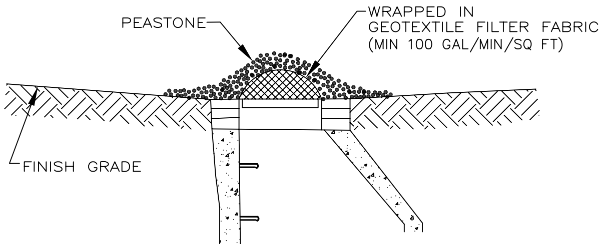
SECTION A-A
